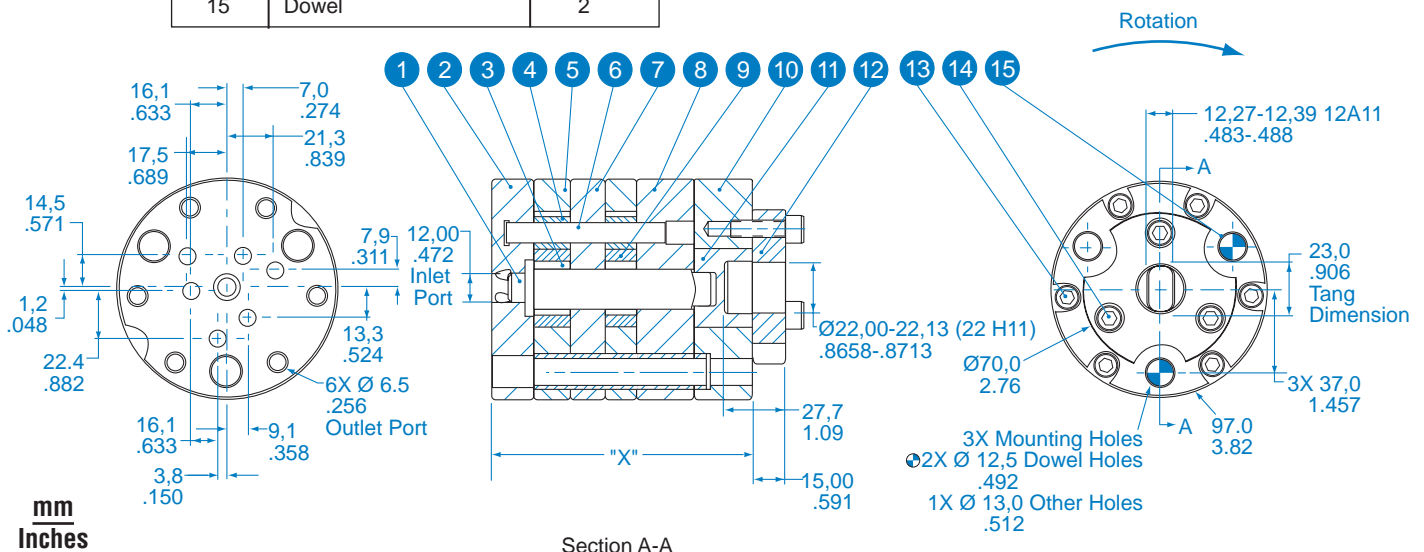
Section A-A
