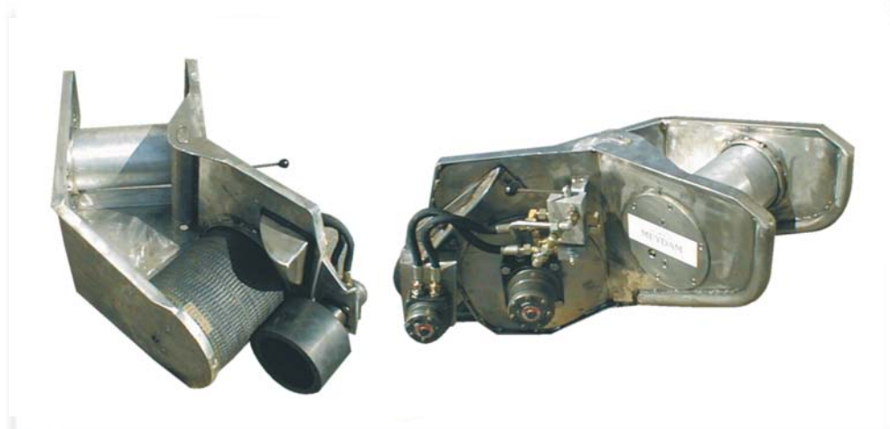
Gillnet haulers 300 kg.
